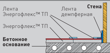
Схема установки тёплого пола
