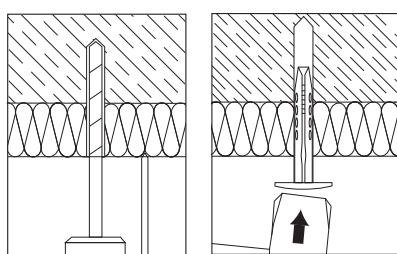
Рисунок 2. Эскиз установки анкера
