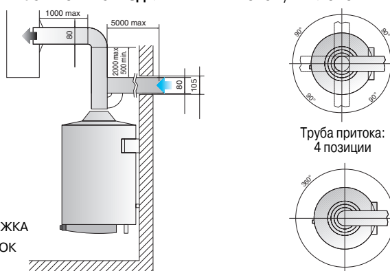
Вытяжная труба: любая позиция
