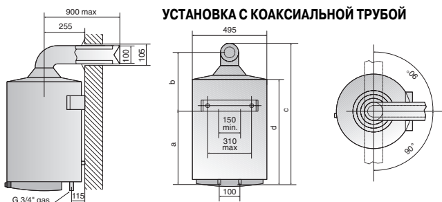
УСТАНОВКА С КОАКСИАЛЬНОЙ ТРУБОЙ
