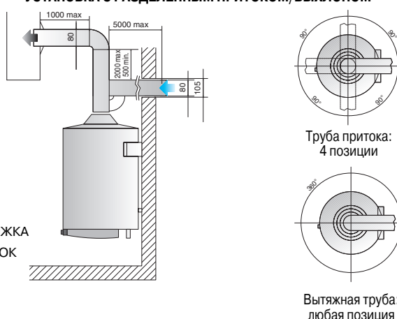
УСТАНОВКА С РАЗДЕЛЕННЫМ ПРИТОКОМ/ВЫХЛОПОМ
